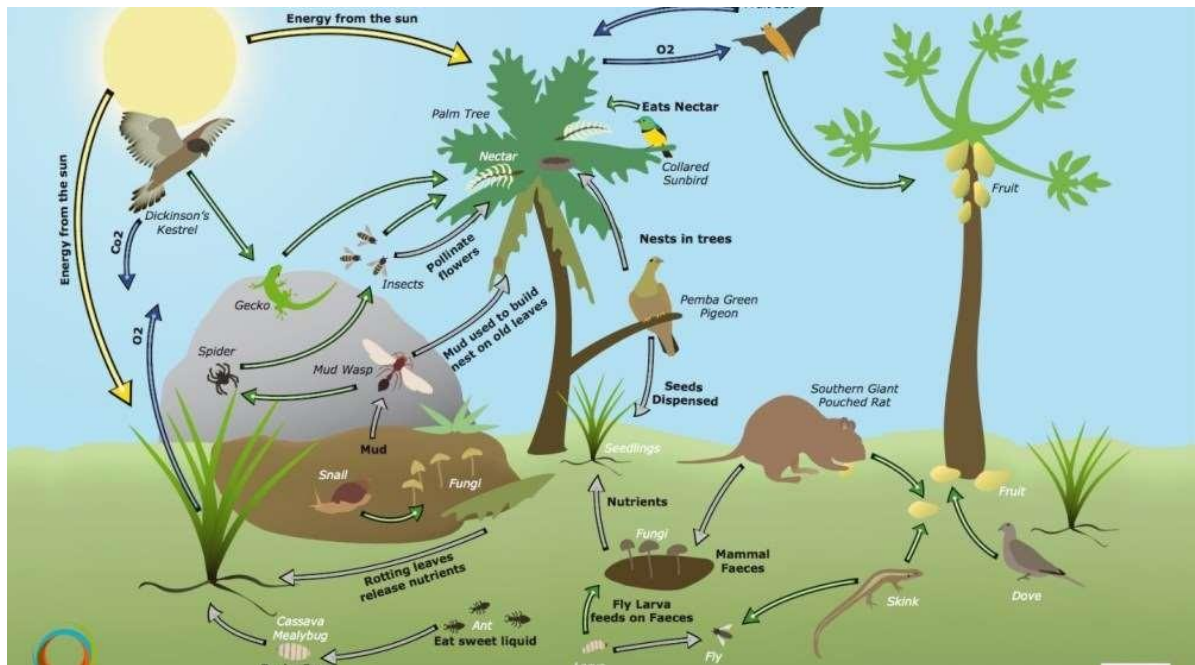
BIODIVERSITY
