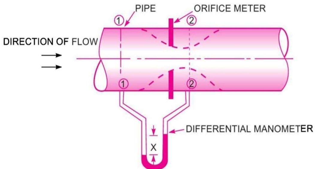
ORIFICEMETER
