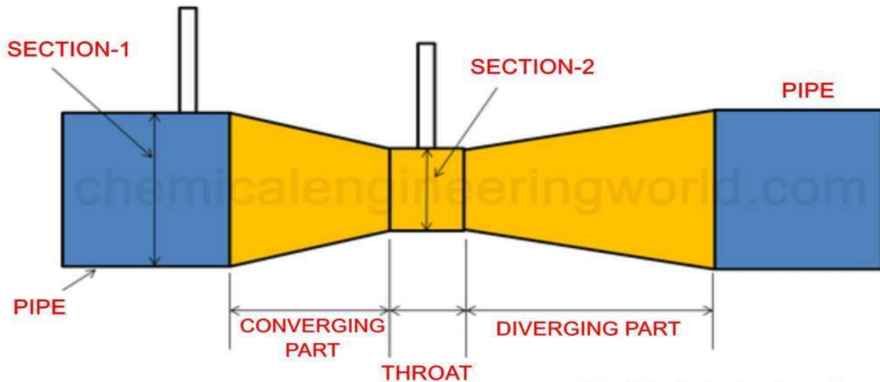
VENTURIMETER
